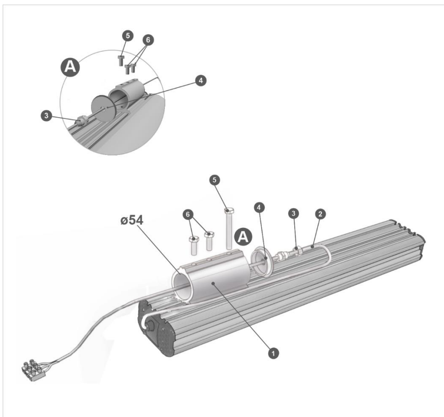
Рисунок 1. Схема монтажа светильника GSTO.
